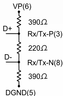
图 5 总线终端器
