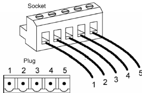
图 3 模块接线图
