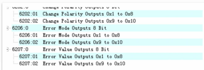
图 9 数字量输出参数
