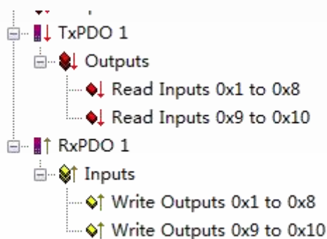
图 6 模块 (R51C1-CAN) 地址映射
