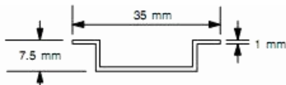
图 2 DIN 导轨
